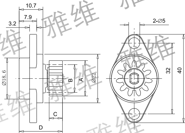
齿轮参数 Gear Specification
